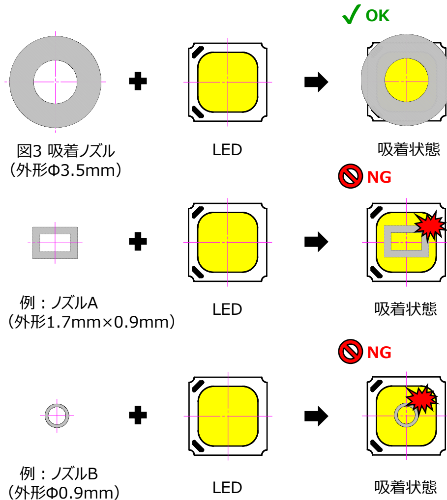
図4. 各種ノズルの吸着例
