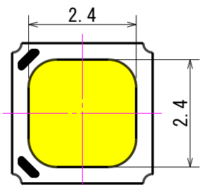
図2. LEDの発光面サイズ
