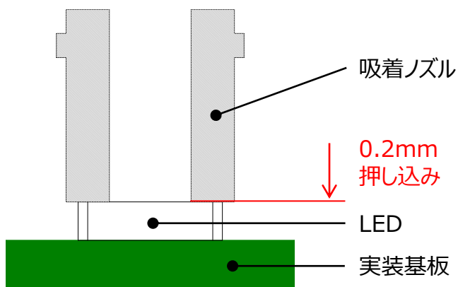
図7. 推奨搭載高さ
