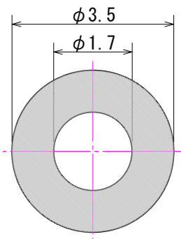
図3. 吸着ノズル先端部形状
